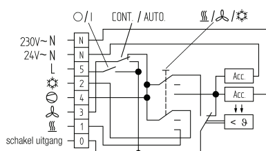
KLR-E 7007
