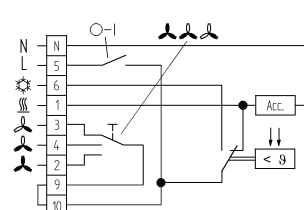
KLR-E 7009
